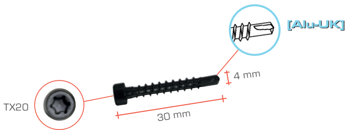
Dazugehörige Spezialschraube für unsichtbaren Abstandhalter für Alu-UK
